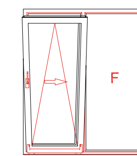
Puerta deslizante paralela
