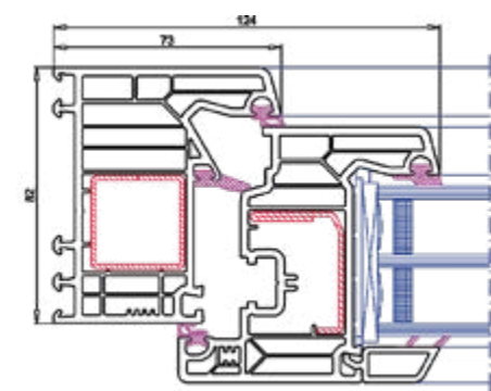
Sección lateral
