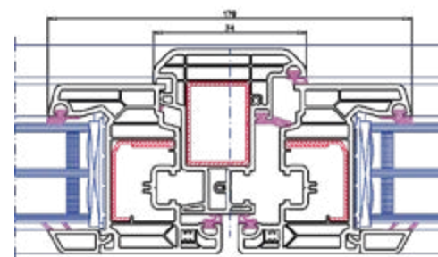
Sección central
