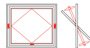
Ventana pivotante
