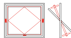
Ventana pivotante
