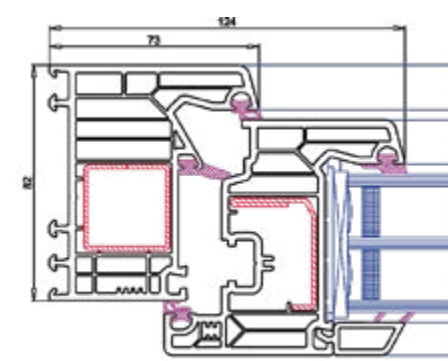
Sección lateral
