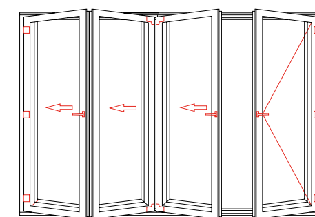
Puerta plegable
