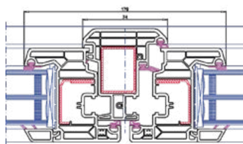
Sección central
