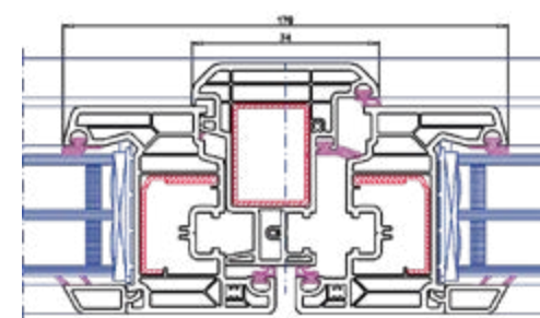
Sección central
